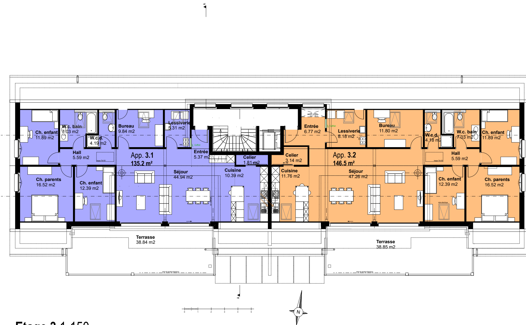
Etage 3 1-150
