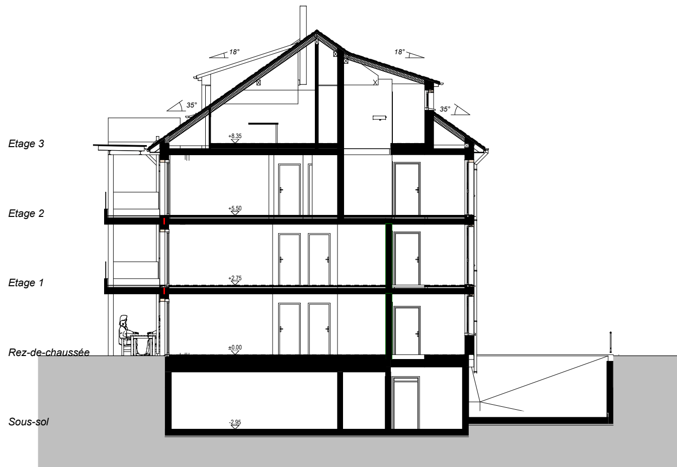
Coupe A-A 1-150
