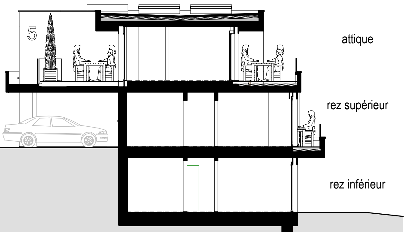
Coupe A-A 1-100
