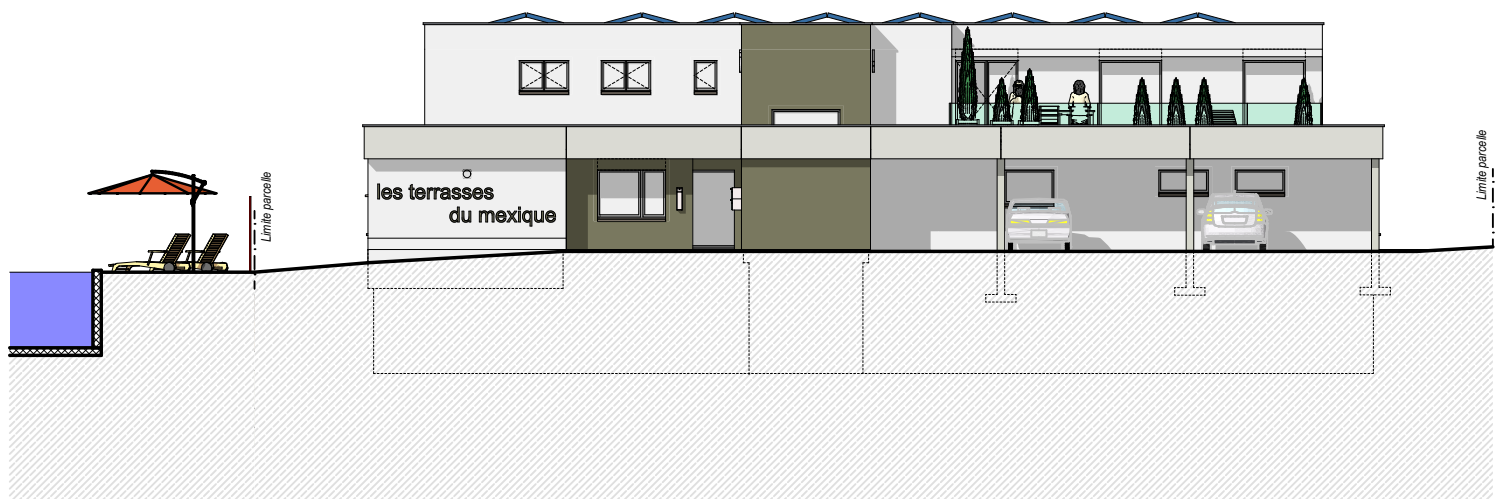
Façade Nord 1-200
